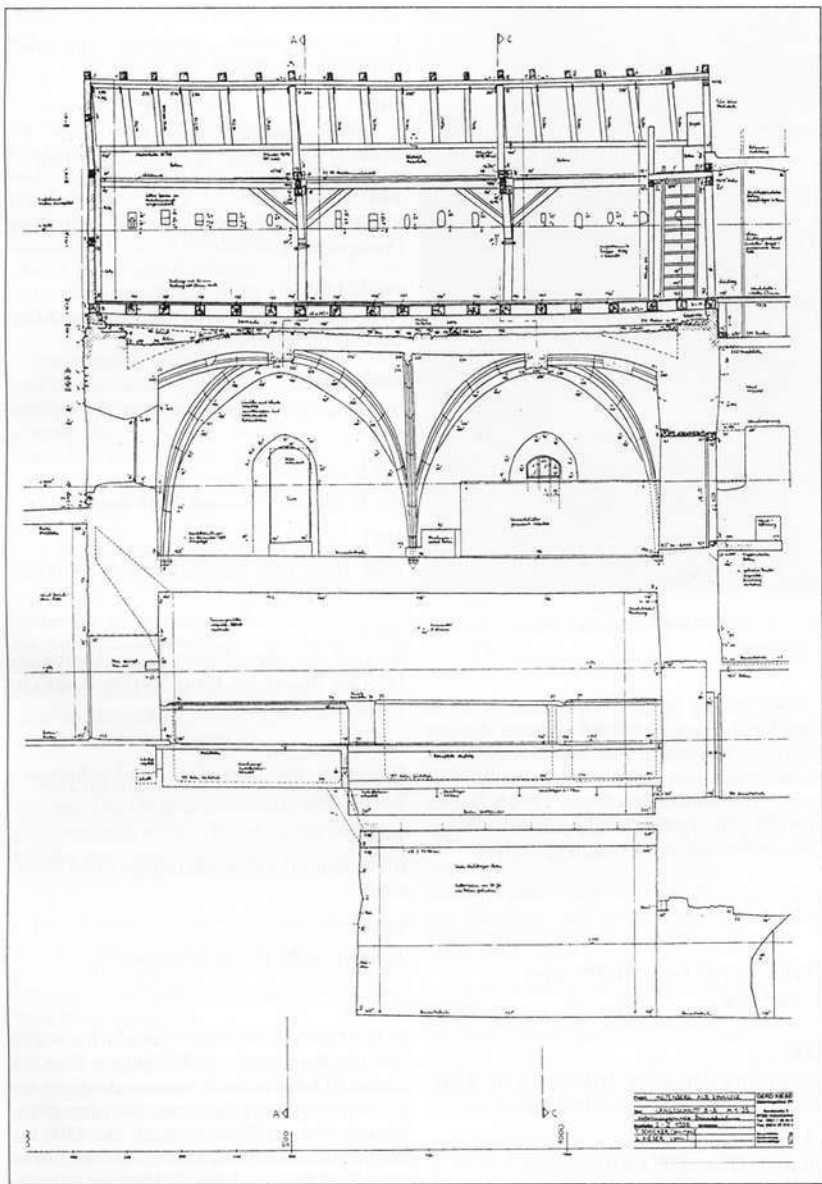
Abb. 6: Längsschnitt B-B mit Blick auf die Südwall.
