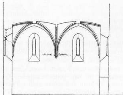
Abb. 64. Miltenberg, Synagoge. Längsschnitt
