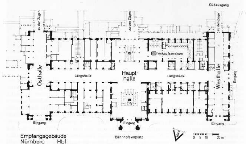
Grundriß Empfangsgebäude 1981
