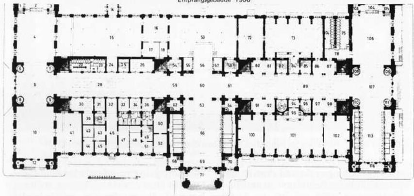
Grundriß des Empfangsgebäudes 1906
