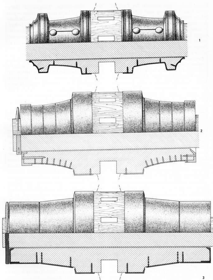
Abb. 14. Rekonstruktion dreier Radnaben. 1 Großesfeld, Lkr. Rhön-Gräberfeld, Gräberfeld 2, Grab 2/1980. — 2 Weinsfeld-Lay, Lkr. Roth, Hügel 4, Grab 5/1976. — 3 Repperndorf, Lkr. Kitzingen, Flur „Am Hügel“, Zentralgrab/1981. — M. 1:3.
