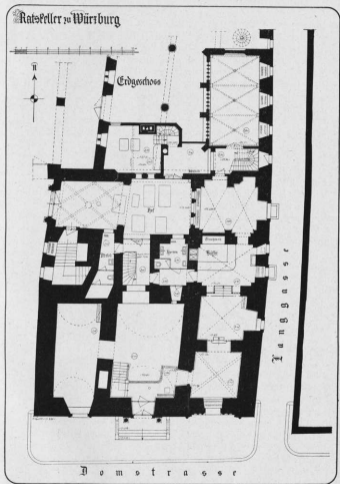
Grundriß des Würzburger Ratstellers (Erdegchoß des Grafen Schardsbaues)
